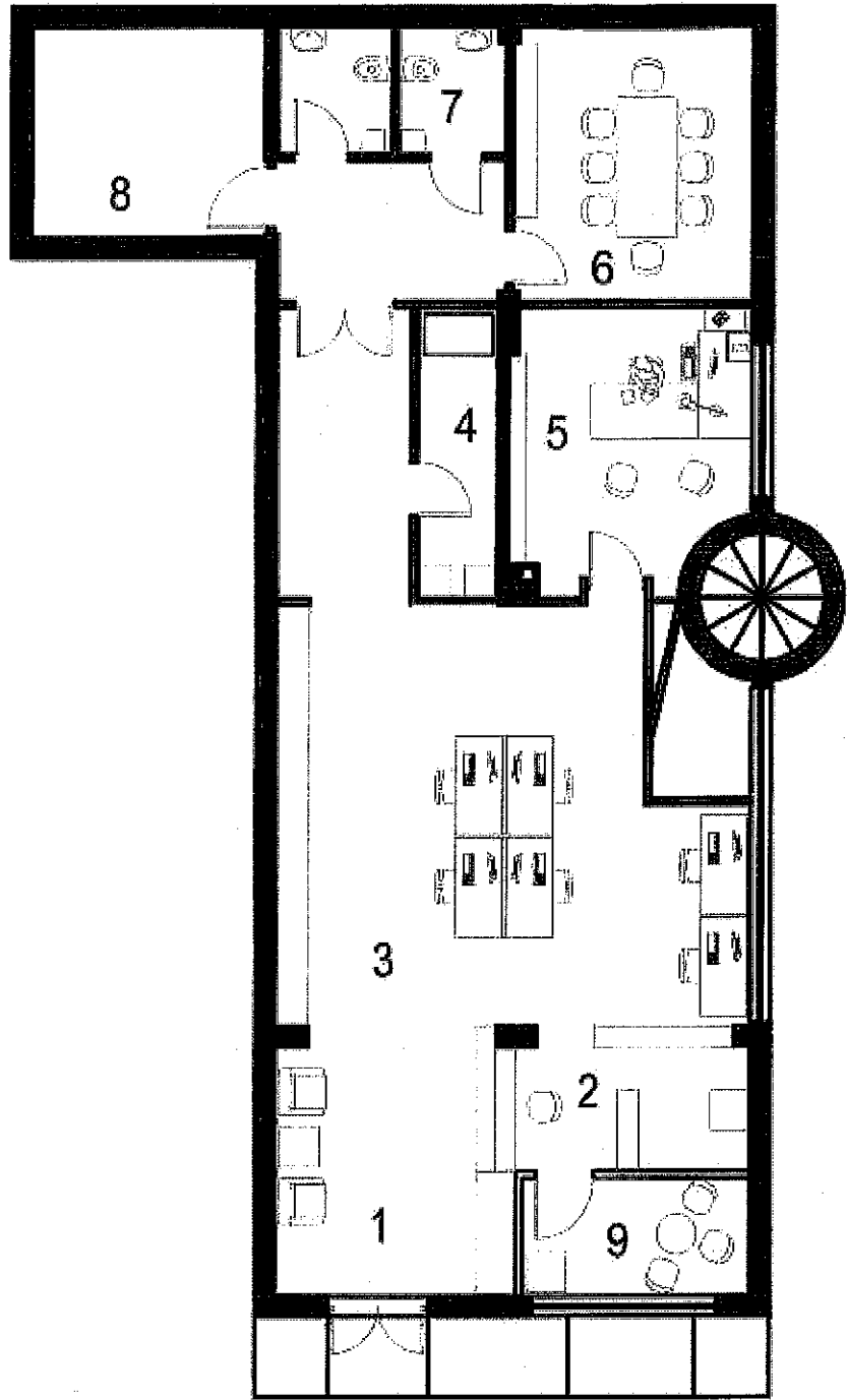
pianta scala 1:200
